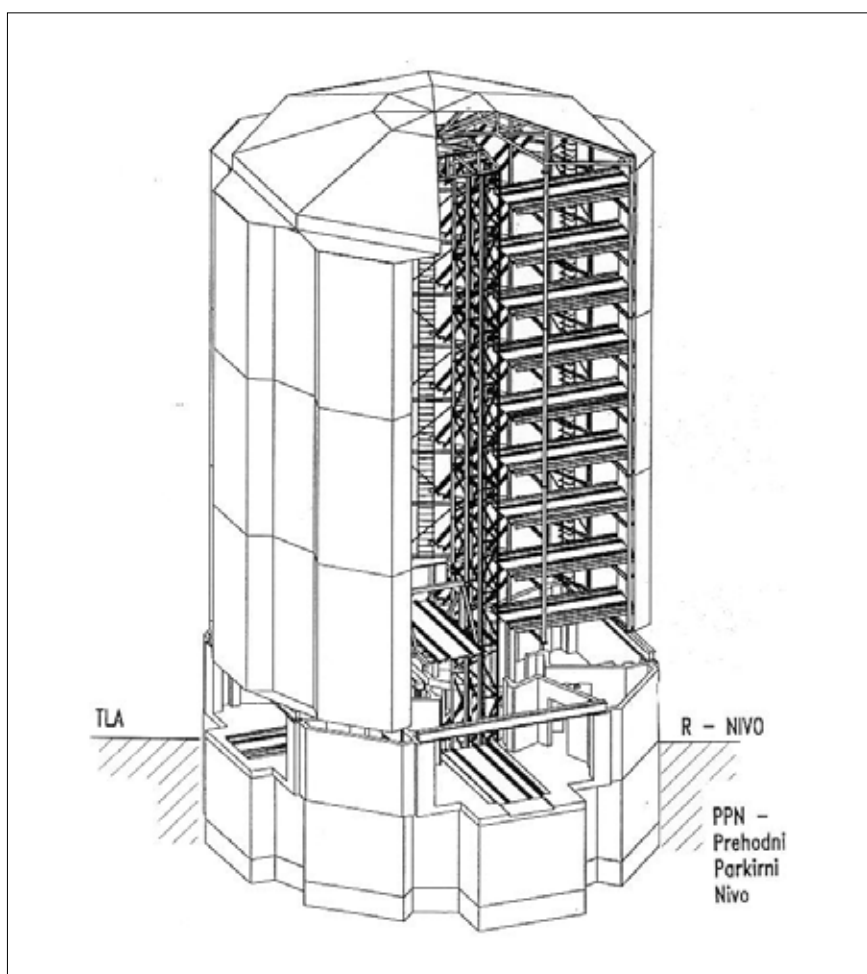
Slika 5. Zasnova avtomatizirane kompaktne garažne hiše COMPA
